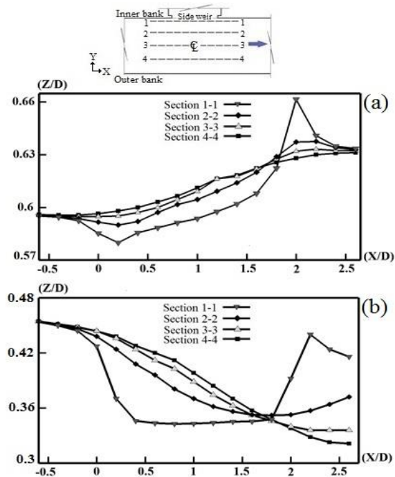
شکل ۸- تراز سطح آزاد آب در حالت سرریز جانبی مستغرق برای مقاطع طولی مختلف (a) جریان زیر بحرانی (b) جریان فوق بحرانی.
