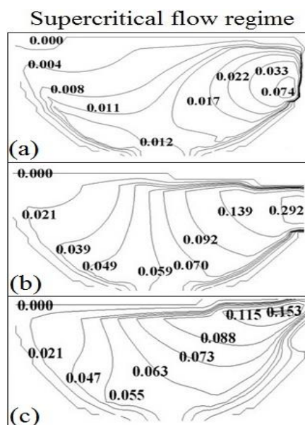
شکل ۹- خطوط هم‌تراز سرعت عرضی در (a) ابتدا (b) وسط و (c) انتهای سرریز جانبی مستغرق برای رژیم جریان فوق بحرانی.
