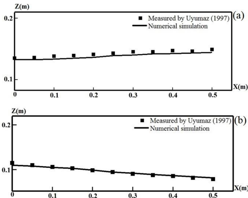
شکل ۲- مقایسه بین نتایج آزمایشگاهی و شبیه‌سازی عددی پروفیل طولی سطح آزاد جریان برای رژیم زیربحرانی (a) رژیم فوق بحرانی (b).
