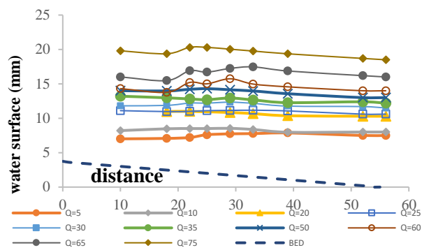
شکل ۴- پروفیل جریان در کانال برای دبی‌های مختلف.
