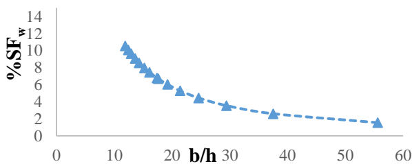
شکل ۱۳- درصد نیروی برشی کل وارده بر دیواره‌ها ( SF_w %) برای نسبت‌های مختلف عرض به عمق ( b/h )
