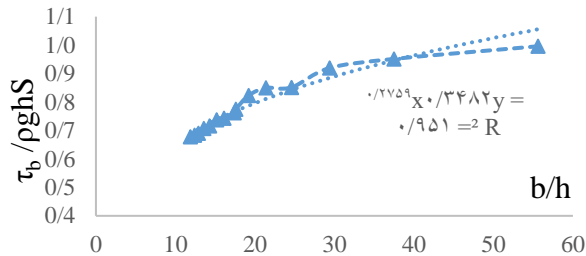
شکل ۱۲- تنش برشی بی‌بعد برای b/h های مختلف.
