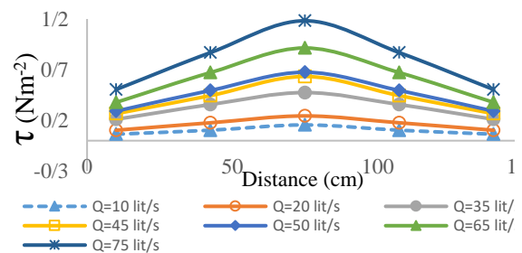
شکل ۱۱- تنش برشی کف برای مقطع عرضی کانال.
