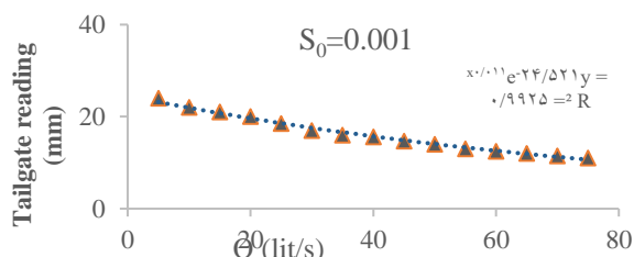
شکل ۵- نمودار دبی - عمق - دریچه پایین دست
