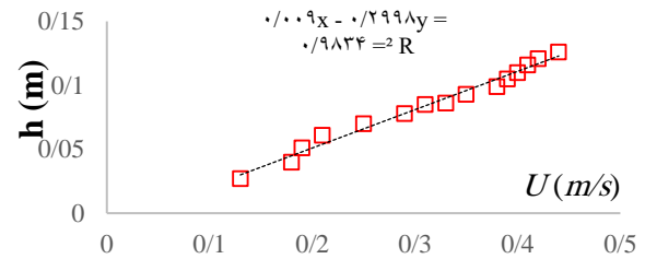
شکل ۱۰- نتایج اندازه‌گیری سرعت میانگین در مقطع OB2
