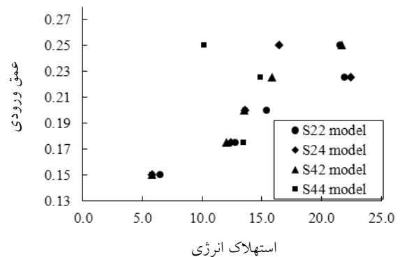
شکل ۷- مقایسه درصد استهلاک انرژی در مدل‌ها
