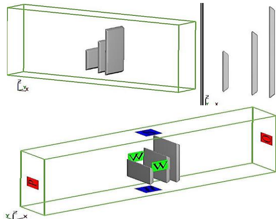
شکل ۲- شبکه محاسباتی و شرایط مرزی اعمال شده برای مدل دریاچه‌های متوالی S_{42} .
