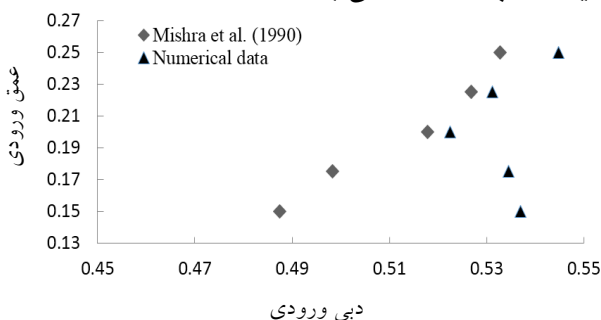
شکل ۳- مقایسه نتایج حل عددی با داده‌های آزمایشگاهی مدل S_{22} .
