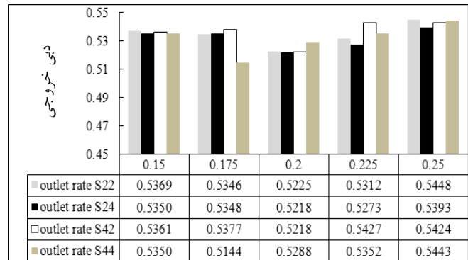
شکل ۶- مقایسه مقادیر دبی خروجی مدل‌ها با یکدیگر.
