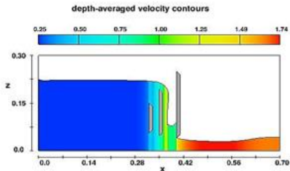
شکل ۴- نمودار دوبعدی تغییرات عمق و سرعت جریان جریان برای مدل با ورودی جریان ۲۲/۵ سانتی‌متر.
