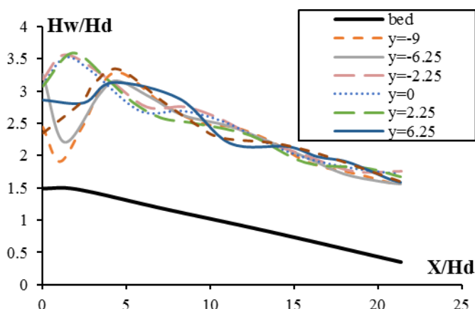
شکل ۱۰- پروفیل سطح آب در دبی ۲۲/۶ لیتر بر ثانیه در زاویه ۹۰ درجه متقارن.
