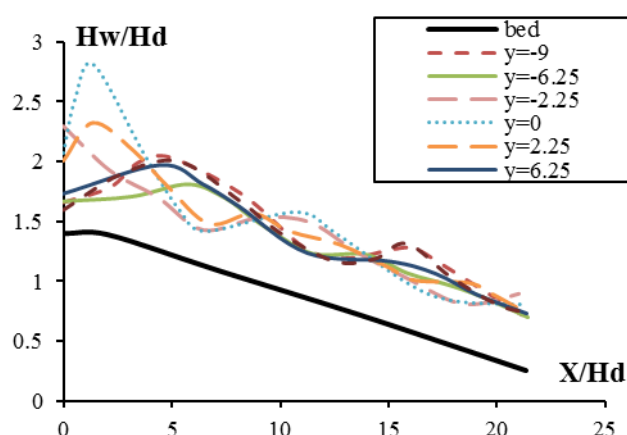
شکل ۹- پروفیل سطح آب در دبی ۵/۶۵ لیتر بر ثانیه در زاویه ۹۰ درجه.
