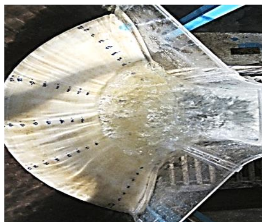
شکل ۱۳- پدیده پرش هیدرولیکی در پنجه سرریز.
