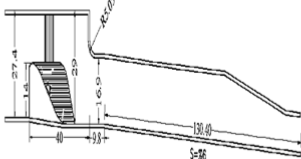
شکل ۲- پیزومترهای کف کانال.
