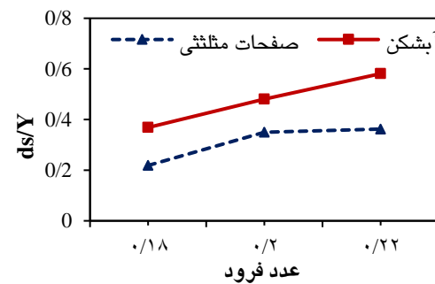
شکل ۷- تغییرات بیشینه عمق آبشستگی در دماغه سازه اول برای صفحات مثلثی و آبشکن‌های مستطیلی به ازای اعداد فرود مختلف.
