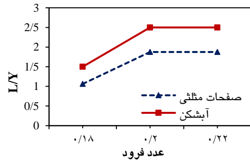
شکل ۵- تغییرات طول چاله آبشستگی در برابر عدد فرود جریان برای صفحات مثلثی و آبشکن‌های مستطیلی.
