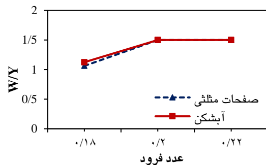
شکل ۶- تغییرات عرض چاله آبشستگی در برابر عدد فرود جریان برای صفحات مثلثی و آبشکن‌های مستطیلی.
