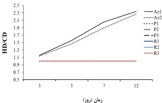
شکل ۳- مقایسه نسبت HD/CD ۸ جدایه در ارزیابی کیفی انحلال فسفات معدنی پس از گذشت ۱۲ روز. جدایه‌های Az1 و Az2 از تو بارور، جدایه‌های R1, R2 و R3 از روئین و جدایه‌های P1, P2, P3 از فسکو بدست آمده‌اند.
