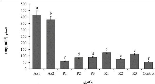
شکل ۴- میزان انحلال فسفات معدنی جدایه‌ها در روش ارزیابی کمی پس از گذشت ۱۲ روز. جدایه‌های Az1 و Az2 از تو بارور، جدایه‌های R1, R2 و R3 از روئین و جدایه‌های P1, P2, P3 از فسکو بدست آمده‌اند.
