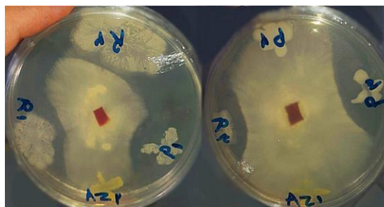
شکل ۷- اثر آنتاگونیستی جدايه‌ها در برابر قارچ بیماریزای فوزاریوم سولانی. جدايه‌هاي Az1 و Az2 از ازتوبارور، جدايه‌هاي R1، R2 و R3 از روئین و جدايه‌هاي P1، P2 و P3 از فسکو بدست آمده‌اند.
