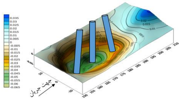
شکل ۸- توپوگرافی سطح بستر در اطراف گروه پایه کج.
