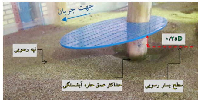
شکل ۵- نمایی از نصب طوقه نامتقارن (3×6) و ۴۰٪
