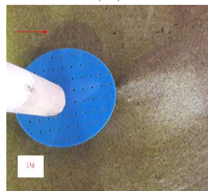
شکل ۱۱- الف) الگوی آبشستگی ب) توپوگرافی بستر با حضور طوقه ۱۵٪ مشبک در فاصله 0.25D از بستر رسوبی.
