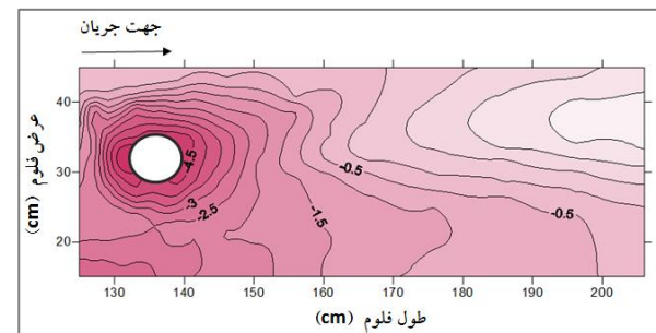
شکل ۸- الگوی آبشستگی در آزمایش شاهد (عدد فرود ۰/۳۷).
