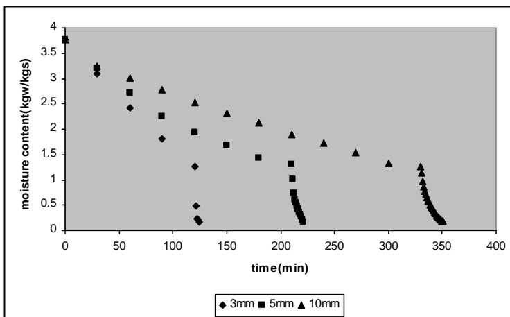
شکل ۴- منحنی زمان خشک کردن برشهای موز با ضخامت های ۱۰، ۵ و ۳ با پیش فرآیند (T 2 )
