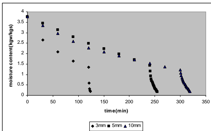
شکل ۵- منحنی زمان خشک کردن برشهای موز با ضخامت های ۱۰، ۵ و ۳ با پیش فرآیند (T 3 )
