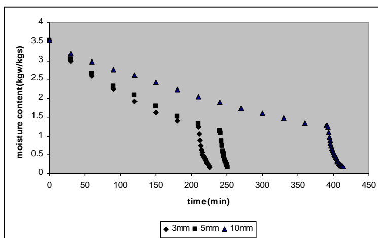
شکل ۴- منحنی زمان خشک کردن برشهای موز با ضخامت های ۱۰، ۵ و ۳ میلی‌متر پیش فرآیند (T1)
