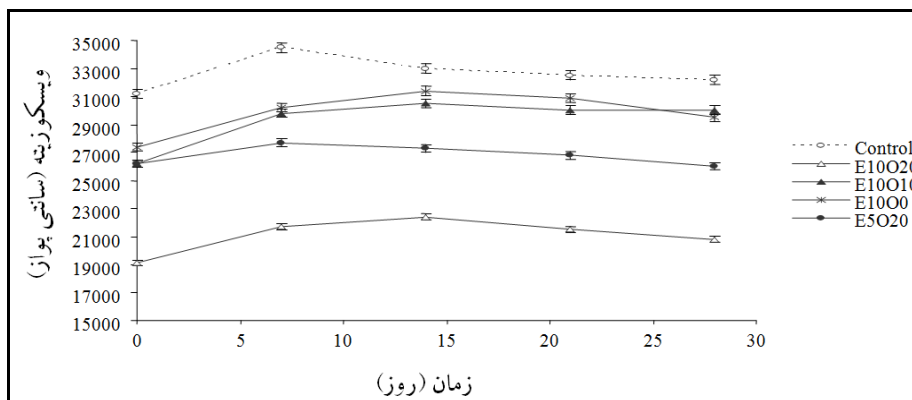
شکل ۶- تغییرات ویسکوزیته در طی نگهداری در نمونه شاهد و غنی شده با فیتواسترول.
