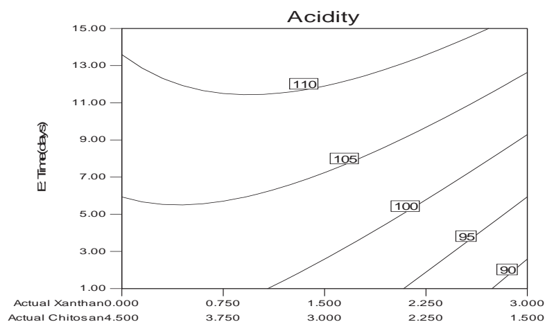
شکل ۱۲- نمودار کانتورپلات اثر نسبت زانتان، کیتوزان و مدت نگهداری بر میزان اسیدیته در مقادیر ثابت اینولین ۹۵/۵ درصد و مقدار کلی صمغ ۱/۵ گرم به ازای ۱۰۰ میلی لیتر شیر
