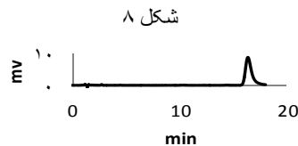
شکل ۴، ۵، ۶، ۷، ۸- کروماتوگرام های سم مورد نظر در غلظت های ۲+، ۷+، ۱۱+، ۱۴+ ppm در شرایط بهینه جداسازی
