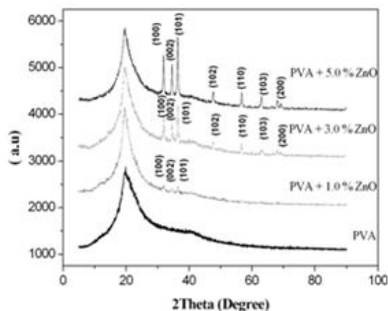
شکل ۳- الگوی پراش پرتو ایکس در پلی وینیل الکل خالص و نانو کامپوزیت های پلی وینیل الکل
