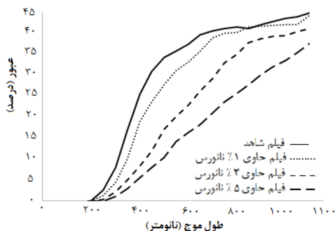
شکل ۵- الگوی میزان عبور امواج طیف UV-Vis فیلم‌های پلی اتیلن ترفتالات حاوی درصد‌های مختلف نانورس.
