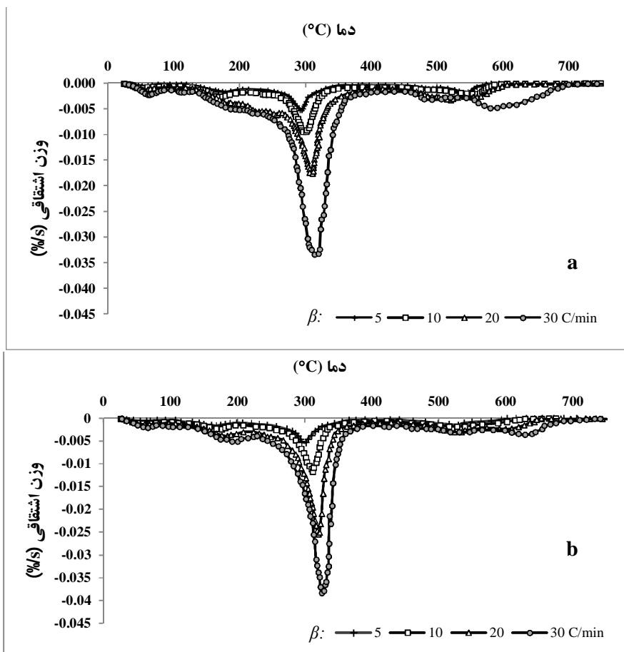
شکل 5- منحنی‌های DTG برای بیوپلاستیک آمیخته (a) و بیوپلاستیک شاهد (b) برای نرخ‌های مختلف گرمادهی (β)
