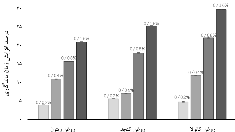
شکل ۴- درصد افزایش زمان ماندگاری (در ۲۵ درجه سانتی‌گراد) تری‌آسیل‌گلیسرول‌های کنجد، زیتون و کانولا در غلظت‌های ۰/۰۲ تا ۰/۱۶ درصد سزامل نسبت به غلظت ۰/۰۱ درصد
