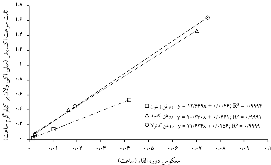
شکل ۵- ارتباط بین معکوس میانگین دوره‌های القاء (غلظت‌های ۰/۰۱ تا ۰/۱۶ درصد سزاملول) و میانگین‌های ثابت سرعت اکسایش تری‌اسیل‌گلیسرول‌های کنجد، زیتون و کانولا در دمای ۶۰، ۸۰ و ۱۰۰ درجه سانتی‌گراد
