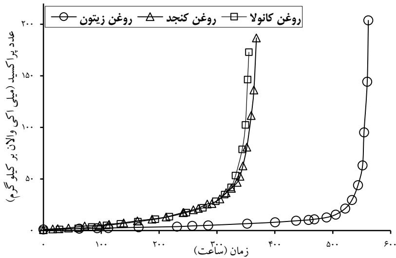
شکل ۳- نمودار سینتیکی اکسایش تری‌اسیل‌گلیسرول‌های کنجد، زیتون و کانولا در غلظت 0.1 \pm 0.1 درصد سزامل و دمای 60 درجه سانتی‌گراد
