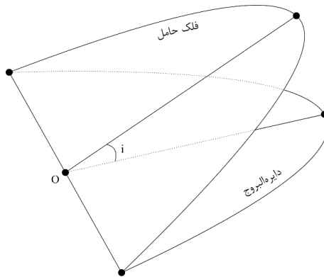
شکل ۴. رأس زاویه میل ( i ) مرکز دایره البروج است (برگرفته از پدرسن، ص ۳۵۷)
