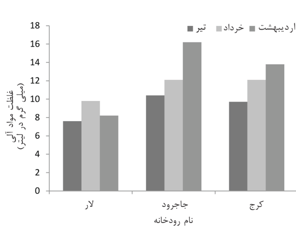
شکل ۳: تغییرات غلظت NOMs در سه ماه نمونه برداری از منابع آب تهران
