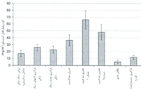
شکل ۴: میانگین تراکم وانحراف معیار گرد و غبار قابل استنشاق در ایستگاه های نمونه برداری فردی
