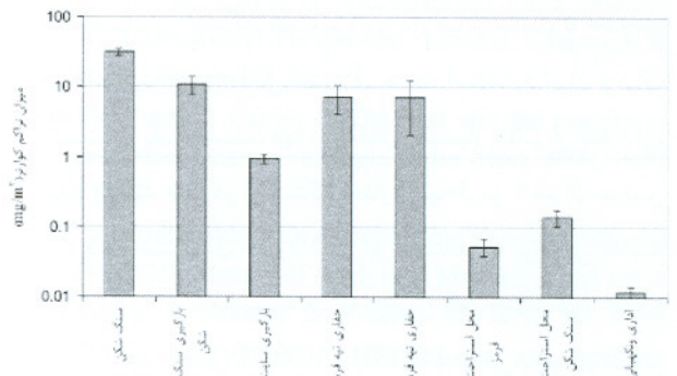
شکل ۳: میانگین تراکم وانحراف معیار کوارتز در گرد و غبار کل در ایستگاه های نمونه برداری کل
