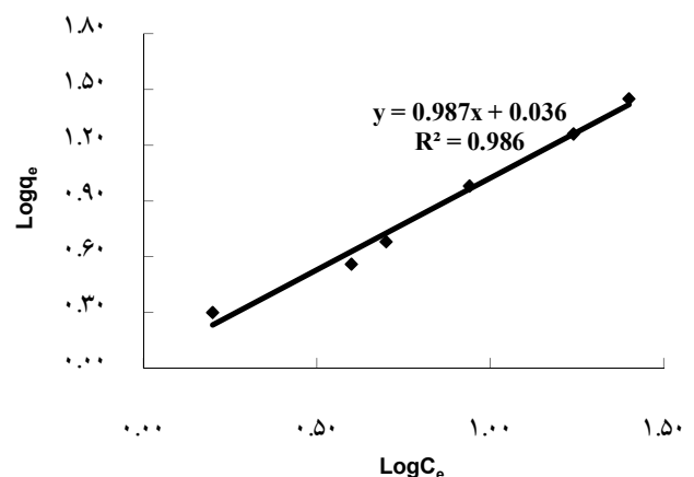
شکل ۸: ایزوترم فروندلیچ در جذب رنگ متیلین بلو با خاکستر استخوان
