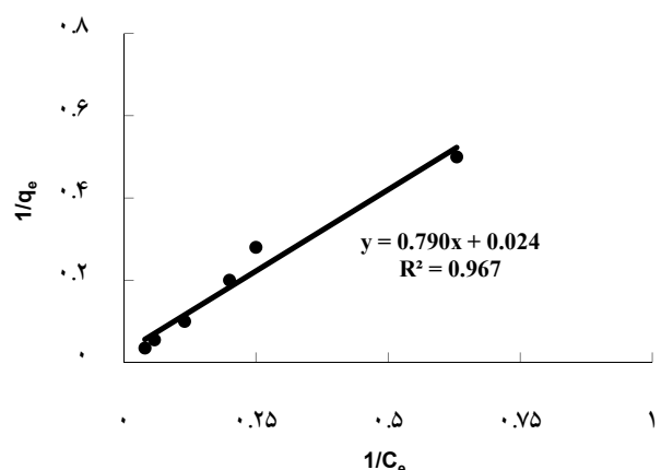
شکل ۹: ایزوترم لانگمیر در جذب رنگ متیلین بلو با خاکستر استخوان
