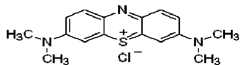
شکل ۱: ساختار شیمیایی رنگ متیلن بلو
