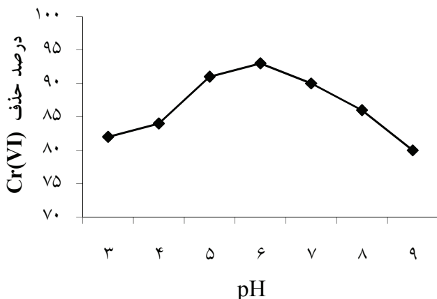
شکل ۳: تأثیر تغییرات pH بر کارایی حذف Cr(VI) در C_{Cr} = 1 \text{ mg/L} و C_{SMZ} = 0.3 \text{ gr}
