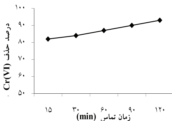
شکل ۴: تاثیر زمان ماند بر کارایی حذف Cr(VI) در C_{Cr} = 1 \text{ mg/L} و \text{pH} = 6 و 0.3 \text{ gr}
