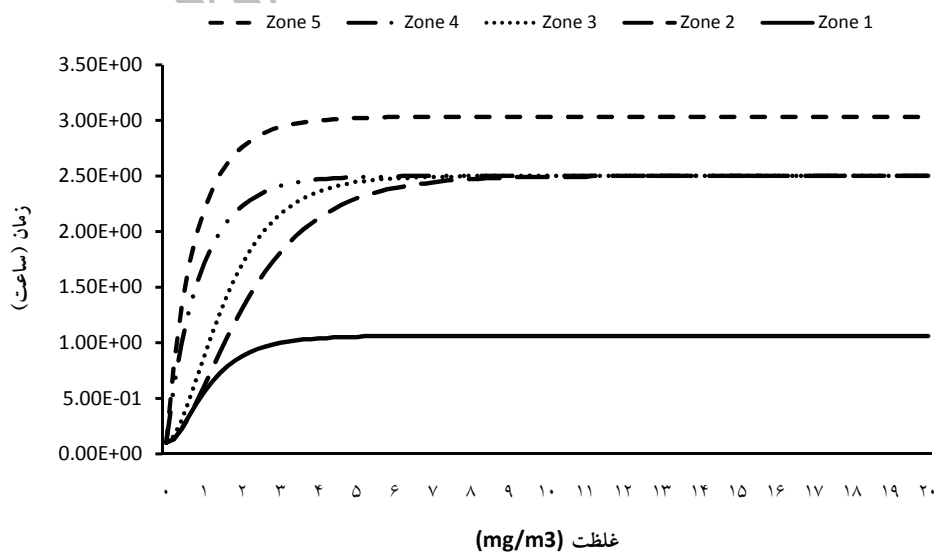
شکل ۳: تغییرات غلظت NO x بر حسب زمان در نواحی مختلف در مدل IAQX 1.0f
