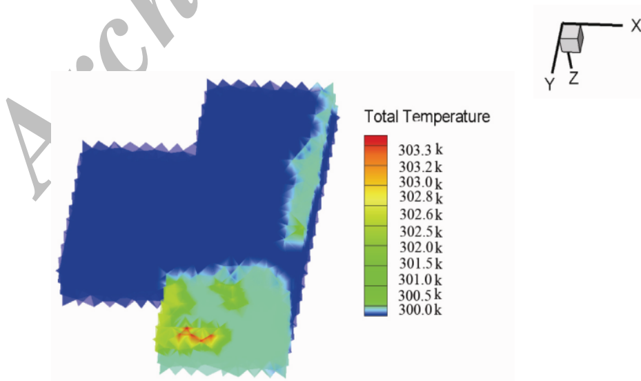
شکل ۶: هم مقدارهای دما در محیط بسته بر حسب کلون
