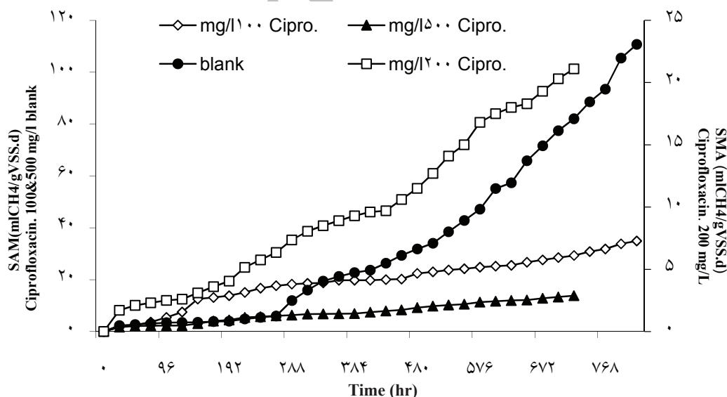
شکل ۲: تاثیر آنتی بیوتیک سیپروفلوکساسین بر روی میزان تجمعی متان سازی ویژه بیومس بی هوازی: (الف): در غلظت های کم شامل، ۱ (▲)، ۰/۱ (○)، ۱ (●)، ۵ (■)، ۵۰ (◊) و شاهد یا صفر (●) میلی گرم در لیتر؛ و (ب) غلظت های زیاد شامل، ۱۰۰ (◊)، ۲۰۰ (◻)، ۵۰۰ (▲)، و شاهد یا صفر (●) میلی گرم در لیتر
