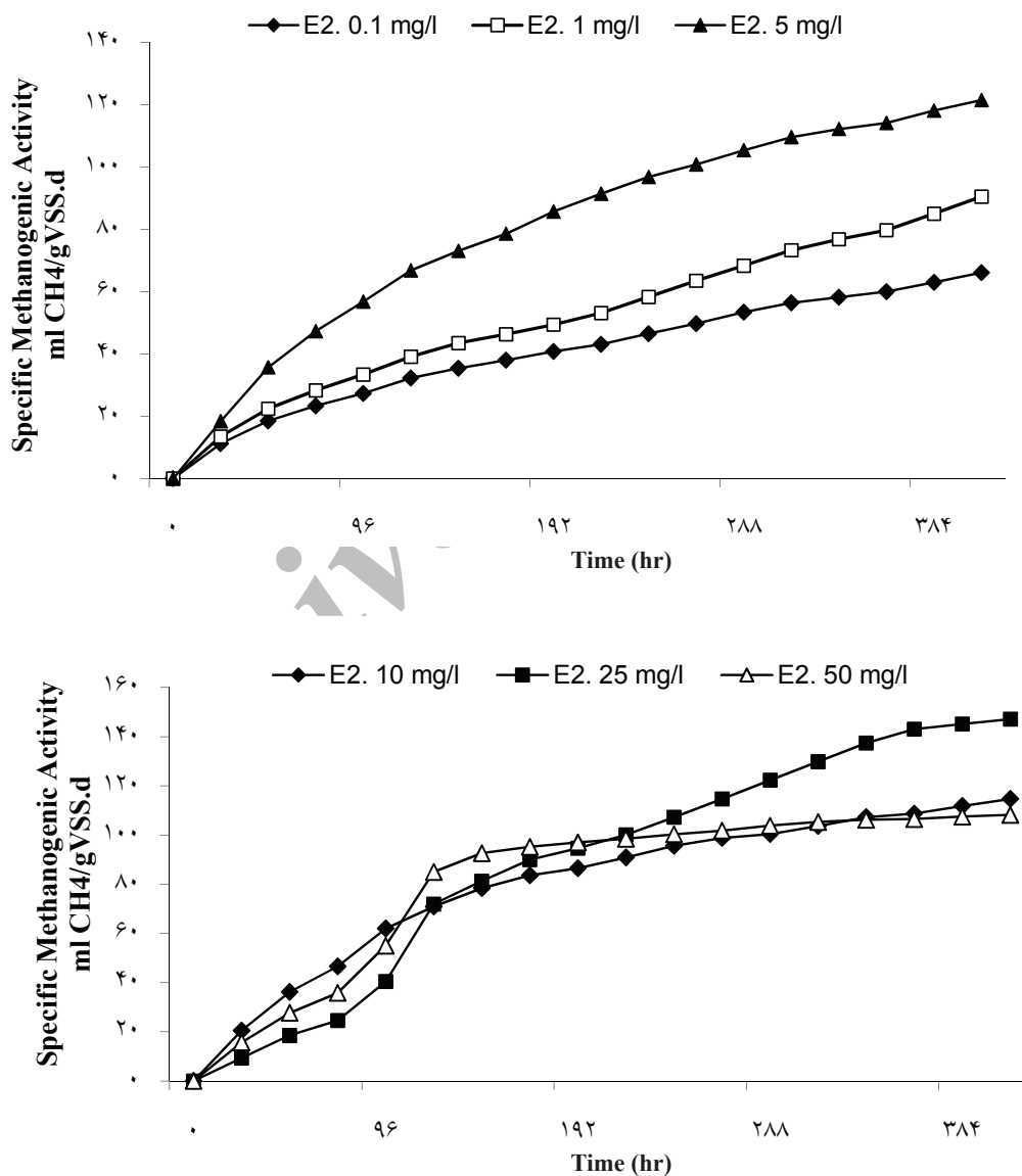
شکل ۴: تاثیر هورمون E2 بر روی میزان تجمعی متان سازی ویژه بیومس بی هوازی: (الف): در غلظت های کم شامل: ۰,۱ (◆)، ۱ (□)، ۵ (▲) میلی گرم در لیتر و (ب) غلظت های زیاد شامل، ۱۰ (◆)، ۲۵ (■) و ۵۰ (▲) میلی گرم در لیتر
