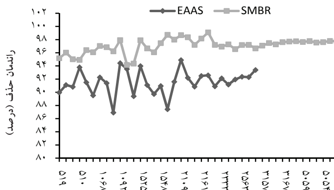
شکل ۳: عملکرد سیستم EAAS و SMBR در حذف COD از فاضلاب سنتتیک غلظت COD ورودی (mg/L)
