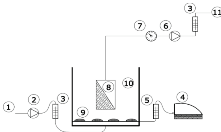
۱- فاضلاب ورودی ۲- پمپ فاضلاب ۳- فلومتر فاضلاب ۴- پمپ هوا ۵- فلومتر هوا ۶- پمپ مکش هوا ۷- گیج فشار سنج ۸- غشای میکروفیلتر ۹- دیفیوزرهای هوا ۱۰- مخزن هوا ۱۱- پساب
