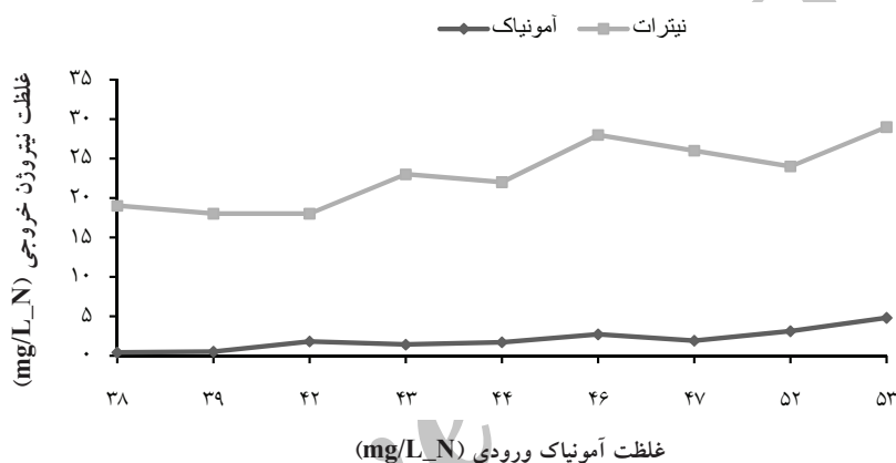
شکل ۶: راندامان حذف نیتروژن و عملکرد فرایند نیتریفیکاسیون در سیستم های EAAS و SMBR
