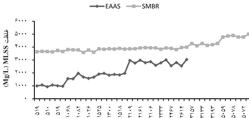
شکل ۲: غلظت MLSS در سیستم های EAAS و SMBR غلظت COD ورودی (mg/L)
