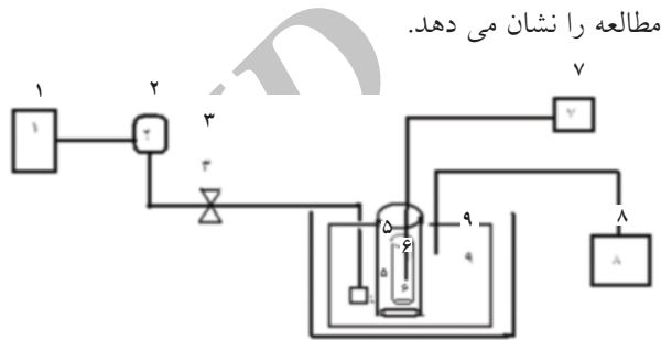
شکل ۱: شمای کلی سیستم پایلوت UV/O_3
