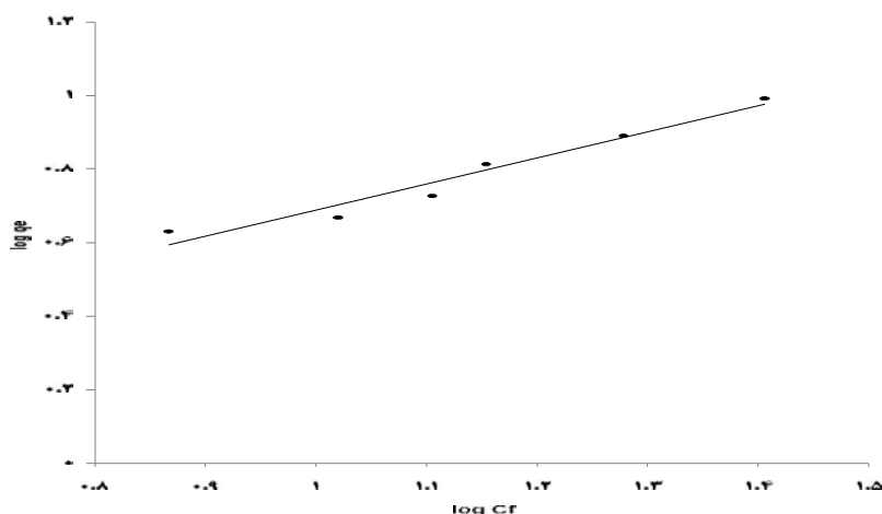
شکل ۸: ایزوترم فروندلیج برای جذب ۴-کلروفنل توسط خاکستر سبوس برنج
