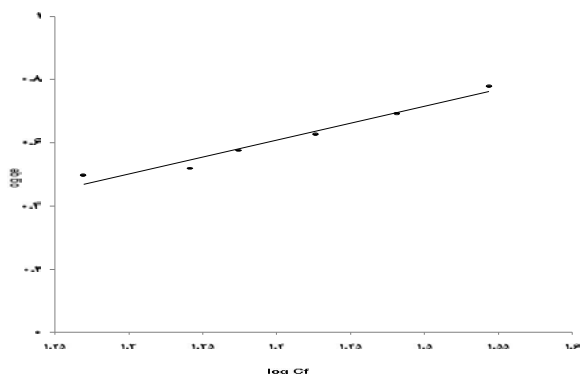
شکل ۷: ایزوترم فروندلیچ برای جذب ۲-کلروفنل توسط
