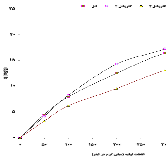
شکل ۳: تاثیر تغییرات غلظت اولیه فنل، ۲-کلروفنل و ۴-کلروفنل بر ظرفیت جذب آنها (زمان تماس ۶۰
