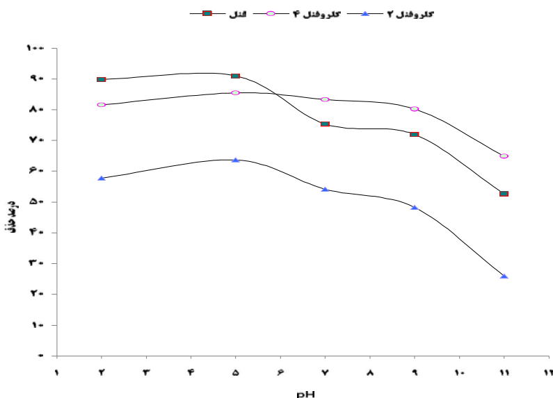
شکل ۲: تاثیر تغییرات pH بر راندمان حذف فنل، ۲-کلروفنل و ۴-کلروفنل (غلظت اولیه ترکیبات فنلی ۵۰ mg/L
