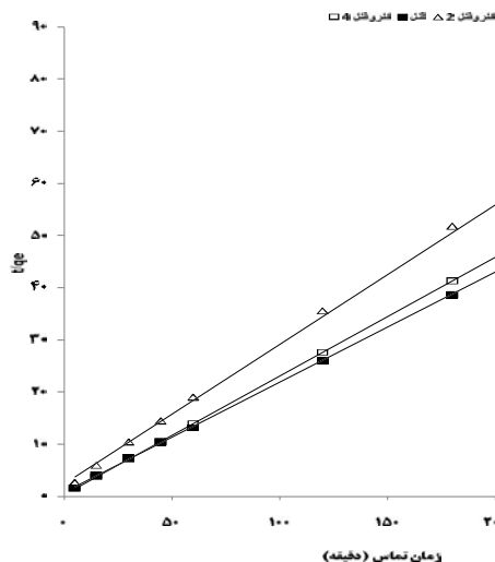
شکل ۵: انطباق داده‌های به دست آمده با مدل شبه درجه دوم
