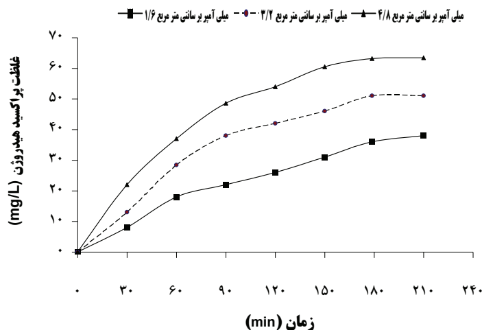
شکل ۷: مقدار پراکسید هیدروژن تولیدی در دانسیته جریان‌های مختلف (pH=3، الکترولیت سولفات سدیم 50 mg/L، هوای ورودی 1/5 L/min)
