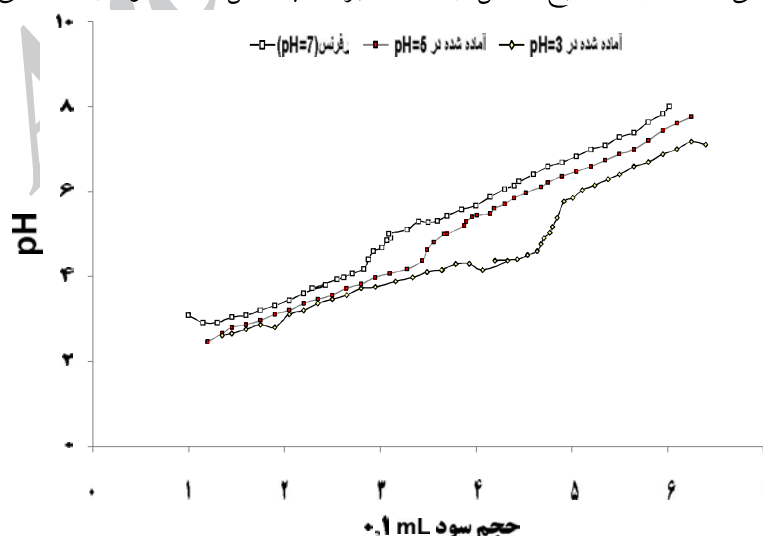
شکل ۳: منحنی تیتراسیون پتانسیومتری نمونه آزلای فعال شده در pH های ۳ و ۵ و ۷ (به عنوان مرجع)
