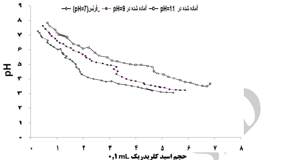
شکل ۲: منحنی تیتراسیون پتانسیومتری نمونه آزلای فعال شده در pH های ۹ و ۱۱ و ۷ (به عنوان مرجع)
