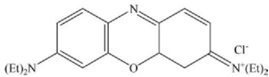
شکل ۱: ساختار شیمیایی رنگینه آبی بازی ۳ ( \lambda_{max} = 654 nm و M_w = 359.9 g/mol)
