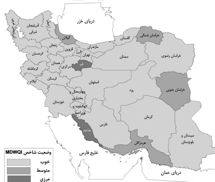
شکل ۱: تصویر کلی کیفیت منابع آب زیرزمینی ایران با استفاده از شاخص MDWQI (میانگین استانی)
