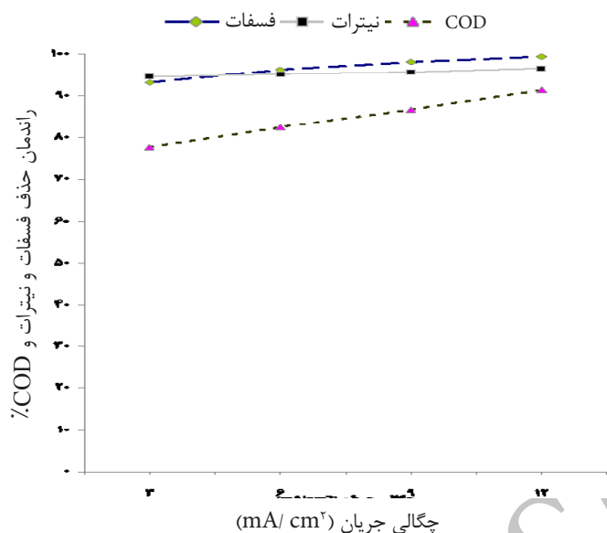
شکل ۷: مقادیر حذف فسفات، نیترات و COD با استفاده از الکترود آهنی و تغییر شدت جریان الکتریکی
