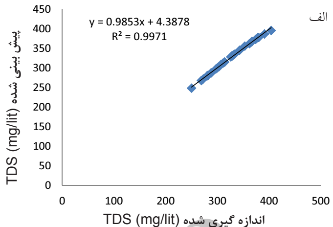
شکل ۹: مقایسه نتایج محاسباتی و مشاهداتی پارامتر TDS رودخانه قره سو کرمانشاه به وسیله (الف) شبکه عصبی مصنوعی و (ب) عصبی مویک
