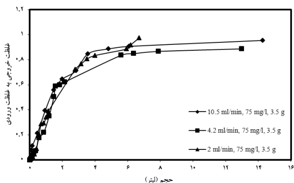
نمودار 5: منحنی شکست بدست آمده از جذب زیستی نیکل توسط جاذب زیستی پروتونه شده C. indica در یک ستون جریان پیوسته با 3/5 g جاذب، غلظت های ورودی 75 mg/L و با نرخ جریان ورودی متفاوت
