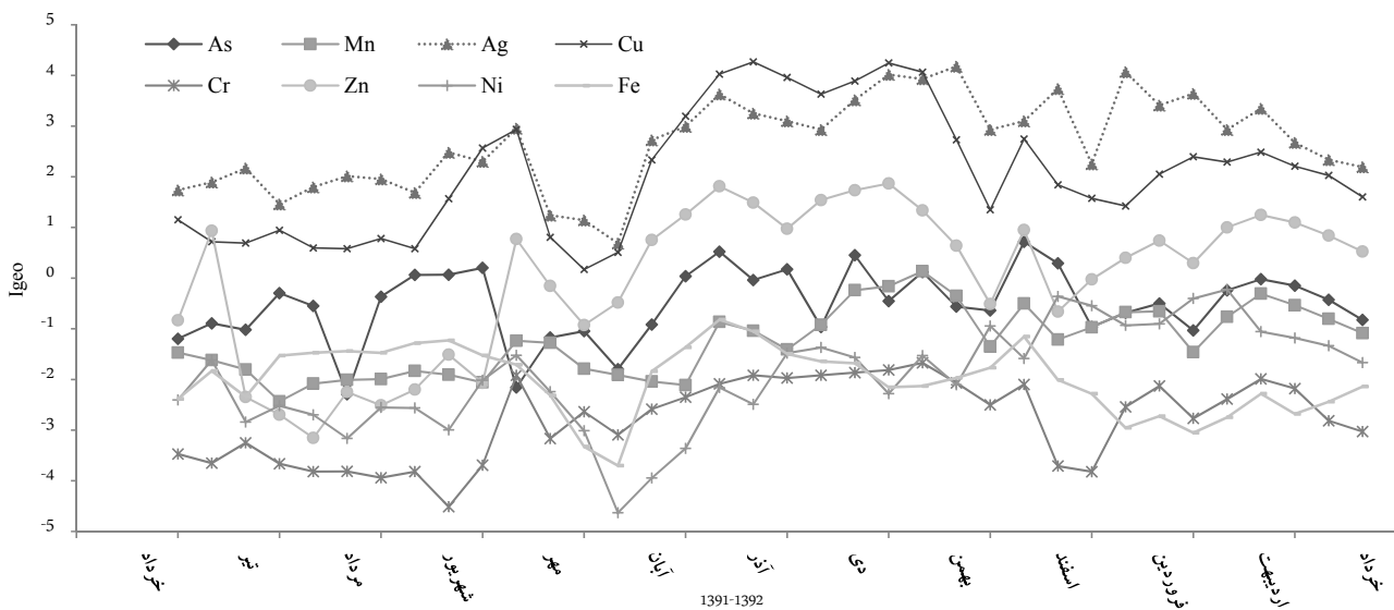
شکل ۳: مقادیر شاخص I_{geo} برای فلزات سنگین اندازه‌گیری شده در ایستگاه سنندج
