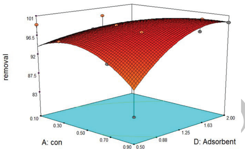
شکل ۶- نمای سه بعدی از راندمان حذف آرسنیک با تغییرات غلظت اولیه و دوز جاذب
