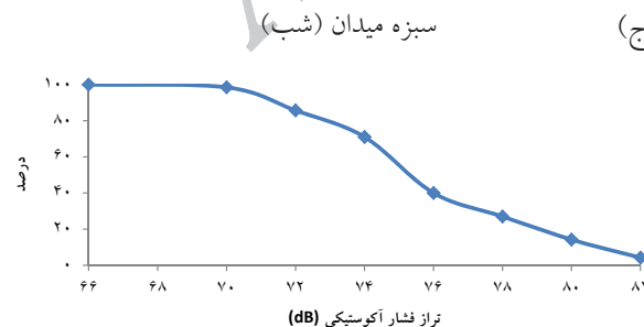
نمودار ۲- منحنی‌های تجمعی مربوط به سبزه میدان، زمستان ۱۳۹۰. (الف صبح ب) عصر ج) شب
