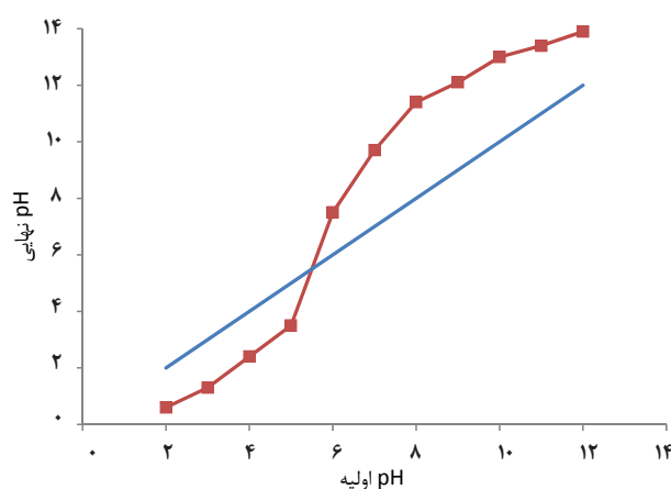
نمودار ۱- تعیین \text{pH}_{\text{zpc}}
