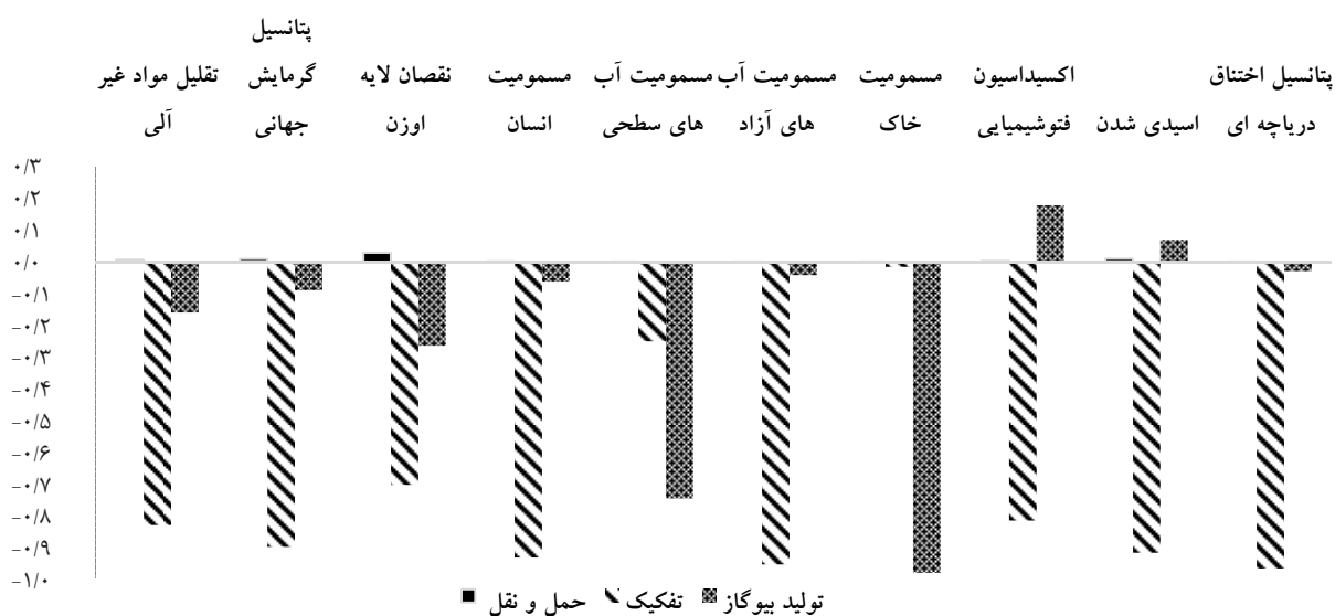
نمودار ۱- سهم هر یک از فرایندها در انتشار و اجتناب از انتشار آلاینده‌های زیستی در زیرسامانه هضم بی‌هوازی
