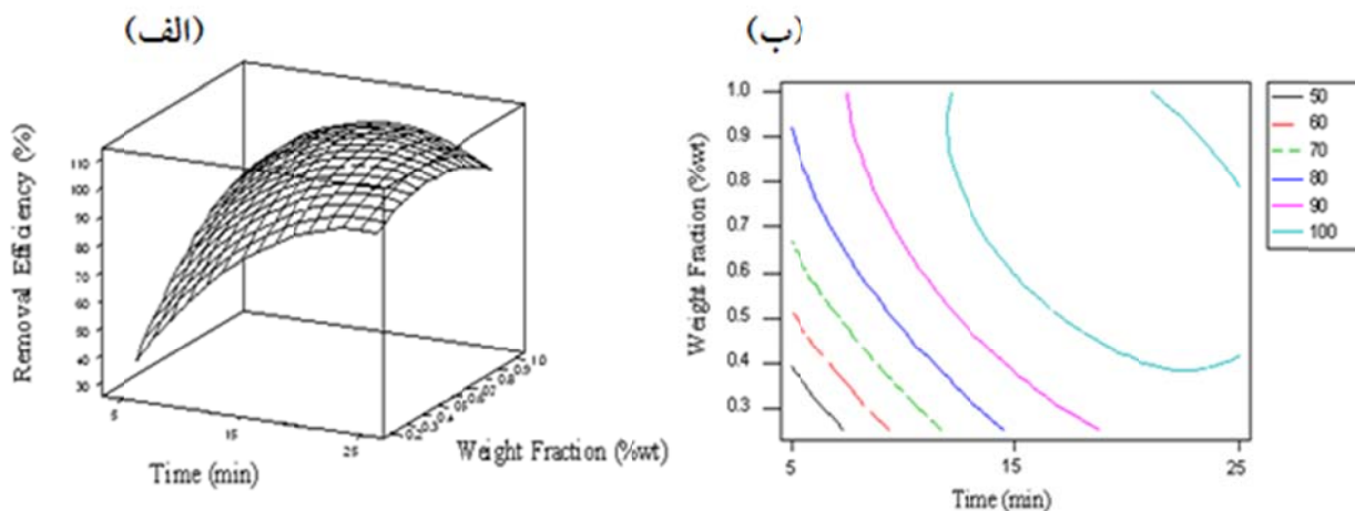
نمودار ۴- الف) پاسخ سطح کارایی حذف آلاینده سوسپانسیون حاوی نانوذرات \text{SnO}_2 نسبت به زمان تابش دهی و غلظت، ب) خطوط کانتور کارایی حذف آلاینده سوسپانسیون حاوی نانوذرات \text{SnO}_2 در زمان تابش دهی و درصدهای وزنی متفاوت
