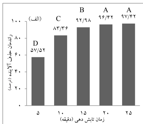
نمودار ۱- الف) تاثیر زمان تابش دهی بر روی میزان فعالیت فتوکاتالیستی محلول حاوی نانوذرات ZnO،
