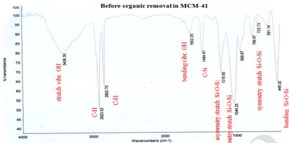
شکل ۱- طیف FT-IR مربوط به ذرات MCM-41 قبل از کلسیناسیون
