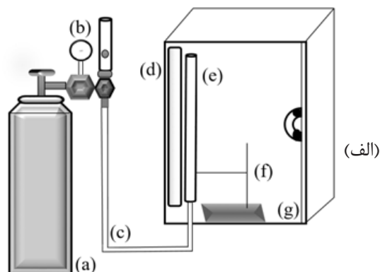
شکل ۱- شمای فتوراکتور (a) کپسول اکسیژن، (b) مانومتر، (c) شیلنگ، (d) لامپ UV-C، (e) راکتور لوله‌ای کوارتز، (f) پایه، (g) محفظه چوبی (الف) و تصویر TEM از نانوذرات TiO_2 (ب)
