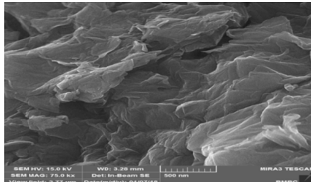
الف) تصویر FESEM اکسید گرافن سنتز شده در مقیاس نانو
