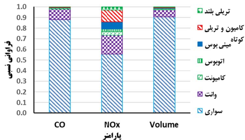
نمودار ۳- تعداد نسبی وسایل نقلیه عبوری در محدوده مورد مطالعه و سهم انتشار وسایل نقلیه در انتشار سالانه CO و NO x در محدوده مذکور
