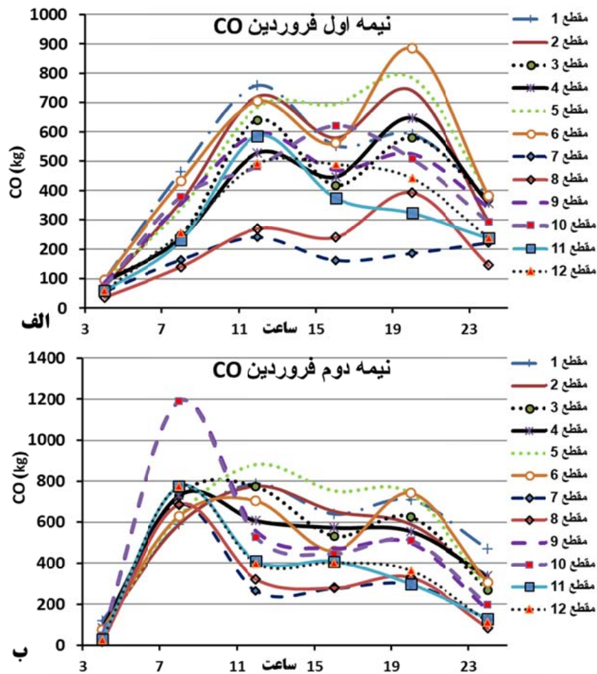
نمودار ۱- تغییرات زمانی کل انتشار CO در روزهای وسط هفته (الف) نیمه اول و (ب) نیمه دوم فروردین ماه
