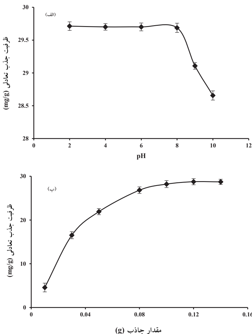
نمودار ۱-الف) اثر pH در مقدار جذب سیلیس بر روی سطح جاذب، ب) اثر مقدار جاذب در مقدار جذب سیلیس بر روی سطح جاذب
