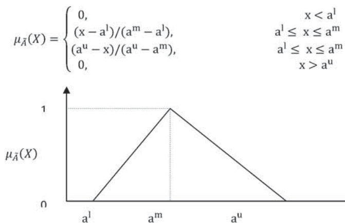
شکل ۲- تابع عضویت و عدد فازی مثلثی [۱۸]
