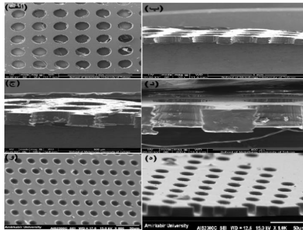
شکل ۲: تصاویر SEM به دست آمده از میکروفیلترهای PDMS، (الف) و (ب) نمای سطح بالا و سطح مقطع جانبی میکروفیلتر ۵۰۰، (ج) و (د) نمای سطح بالا و سطح مقطع جانبی میکروفیلتر ۱۰، (و) و (ه) نمای سطح بالا و سطح مقطع جانبی میکروفیلتر ۱۰
