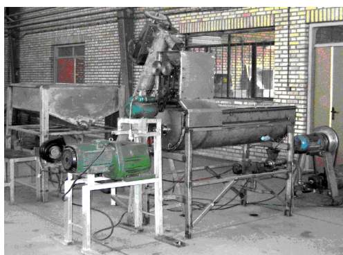
شکل ۱- خط فرآوری روغن زیتون
