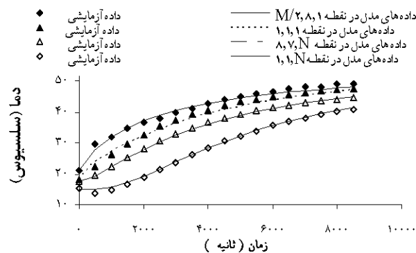
شکل ۶ - مقایسه پروفیل دماهای آزمایشی و داده های پیش بینی شده توسط مدل در نقاط مختلف قوطی در دمای ۵۰ درجه سلسیوس
