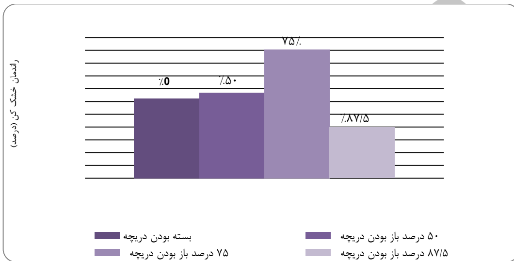
شکل ۶. راندمان خشک‌کن در جریان هوای ۰/۰۱۸ متر مکعب بر ثانیه
