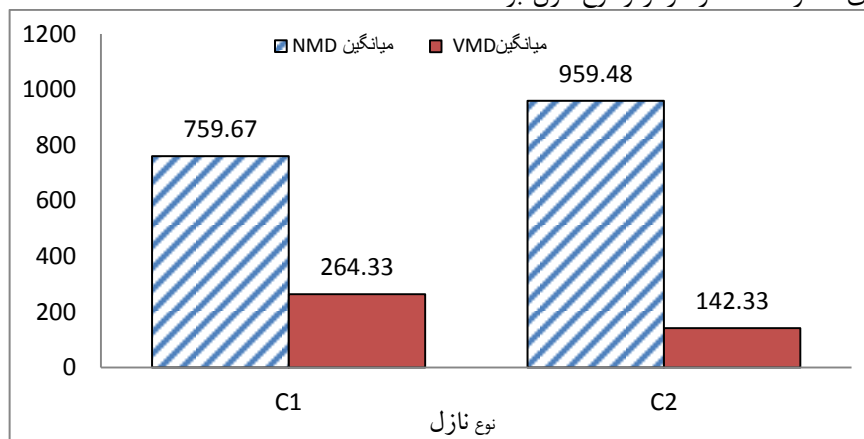
شکل ۶. مقایسه میانیگین اثر نوع نازل بر روی قطر میانه حجمی و قطر میانه عددی
